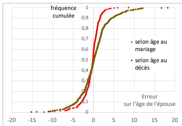
Figure. 6.4. Fonction de répartition de l'erreur sur l'âge au mariage de l'épouse (1668-1792)
