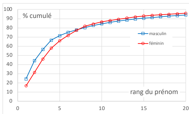
Figure 5.3. Concentration des prénoms masculins et féminins à Trizac : pourcentage cumulé des prénoms à partir du plus fréquent
