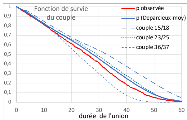
Figure 7.3. Probabilité de survie des couples selon la durée de l'union : comparaison de la loi observée et des simulations avec la table de mortalité de Deparcieux (3 couples d'âges différents et population moyenne)
