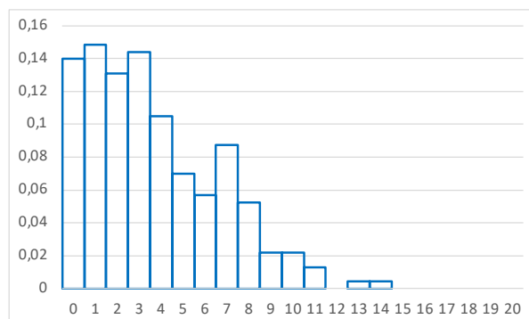
Figure 7.6. Distribution de la taille des familles (229 familles incomplètes)
