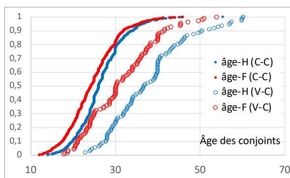
Figure 7.1. Répartition des âges des époux : unions entre célibataires (C-C) et unions entre un veuf et une célibataire (V-C)
