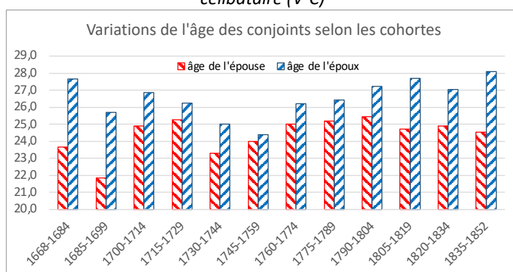
Figure 7.2. Évolution de l'âge moyen au mariage, pour les hommes et les femmes (couples C-C seulement)
