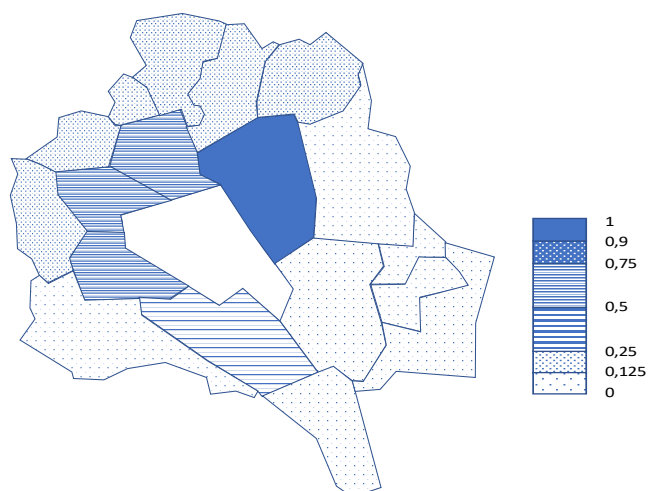
Figure 7.12. Provenance des hommes mariés et établis à Trizac [E-T-T] – 374 cas
