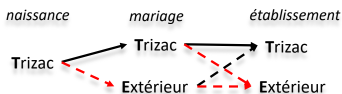
Figure 7.11. Les quatre trajectoires possibles pour les individus nés à Trizac (traits rouges pour les individus qui sortent du corpus, traits noirs pour les individus restant dans le corpus ou y entrant après mariage, traits continus pour les individus non mobiles)
