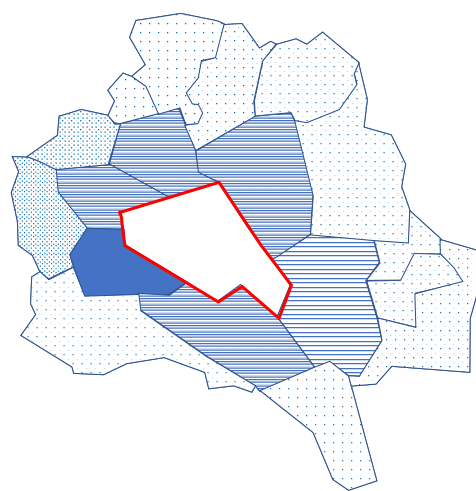
Figure 7.13. Provenance des femmes mariées ailleurs et établies à Trizac [T-E-T]- 253 cas
