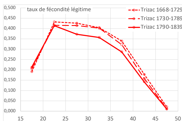
Figure 7.4. Taux de fécondité légitime à Trizac (familles complètes, trois cohortes)
