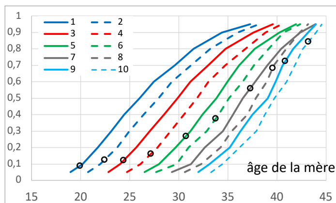
Figure 7.8. Distribution statistique de l'âge des mères pour différents rangs des naissances (figurés circulaires pour la trajectoire du couple Antoine Galvaing x Marguerite Fenolhac)
