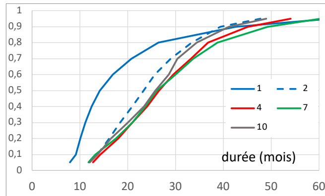
Figure 7.7. Distribution statistique des intervalles : protogénésique (1) et intergénésiques (avant les naissances de rangs 2, 4, 7 et 10)
